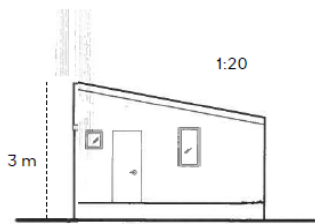
Facadeopstalt; ensidet hældning
